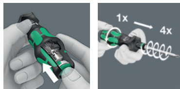
Levering zonder bit
